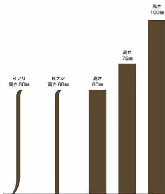
無地巾木・木目巾木実寸図/高さ見本
