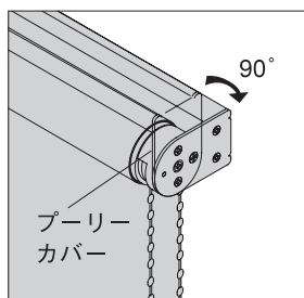
3) プーリーカバーを90°回転させる
