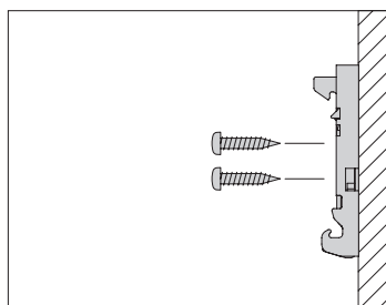
正面付け(窓枠を覆う場合)
