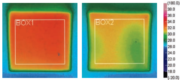
参考写真 サーモグラフィによる熱比較写真 レフランプによる熱照射 20 分後の比較写真 (50216) 左: 50216 コーティング未加工品 右: 50216 コーティング (アルミ) 加工品
