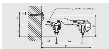
ダブル正面付け (ブラケット幅: 18)
