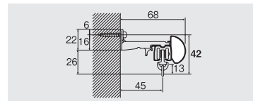
シングル正面付け
