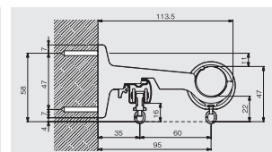
ダブル正面付け (ブラケット幅: 25)
