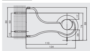
シングル正面付け (ブラケット幅: 32)
