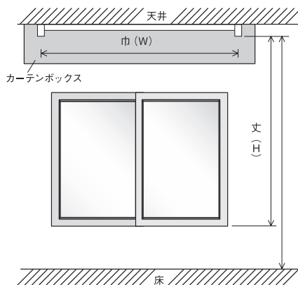
カーテンボックスに取付ける場合
