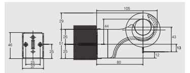
シングル正面付け
