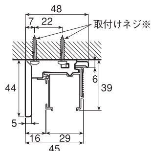
出窓ブラケット天井付け
