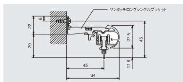
シングル正面付け (ブラケット幅: 18)
