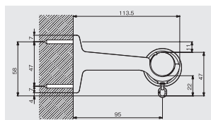
シングル正面付け (ブラケット幅: 25)
