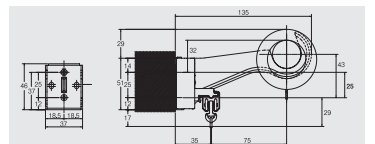
ダブル正面付け
