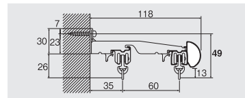
ダブル正面付け
