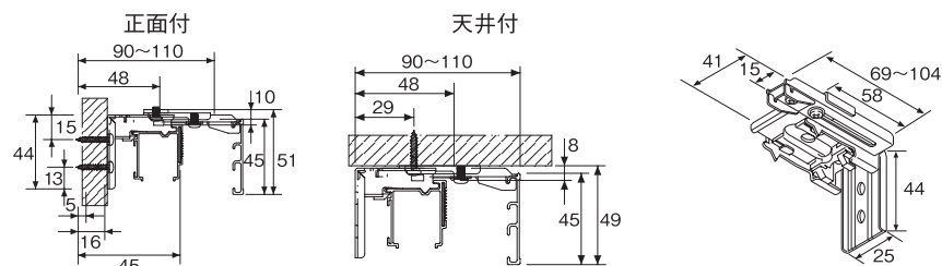
ブラケット寸法図
