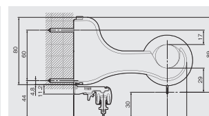
ダブル正面付け (ブラケット幅: 32)
