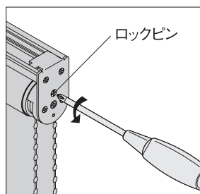
2) ロックピンを解除する
